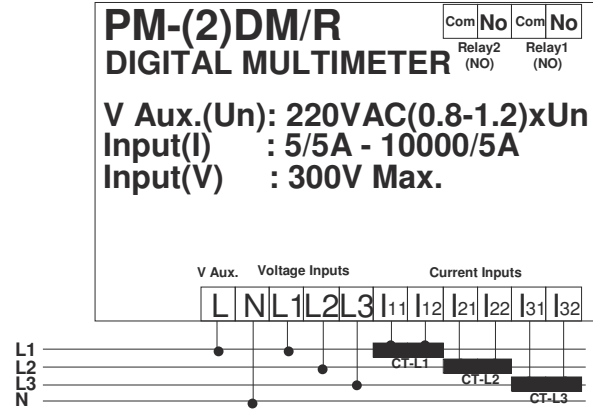
Şekil -1 Bağlantı Şeması
