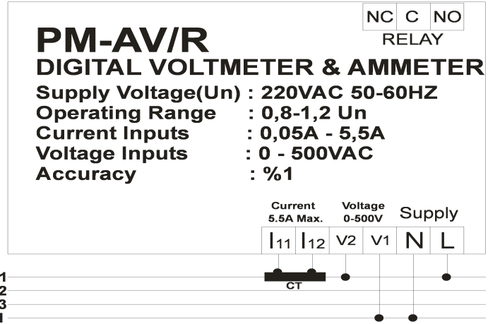
Şekil -1 Bağlantı Şeması
